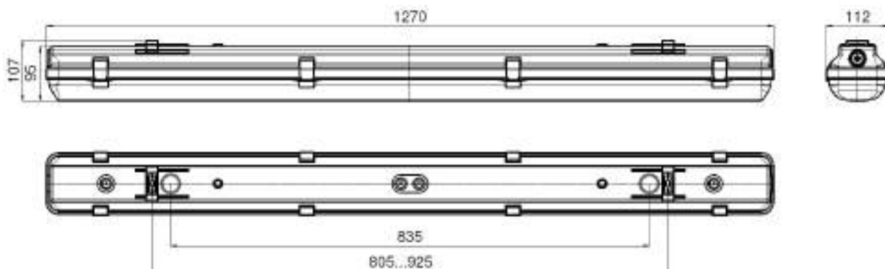
Рис. №2 Габаритный чертёж.
